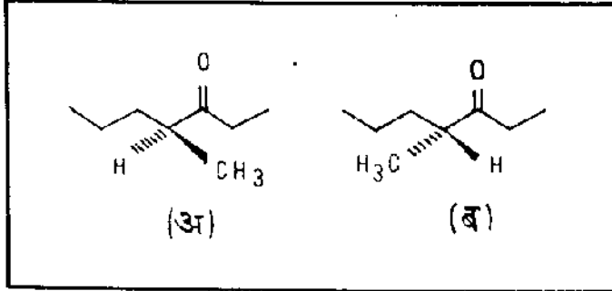
१७. त्रिमितीय समघटक : प्रतिबिंबासारखी संरचना
